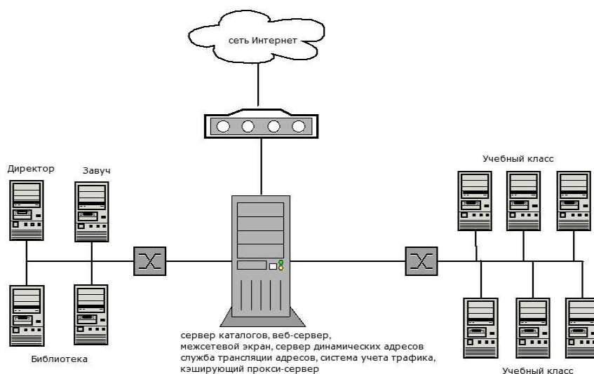
Рис. Схема локальной сети по типу «клиент-сервер»
